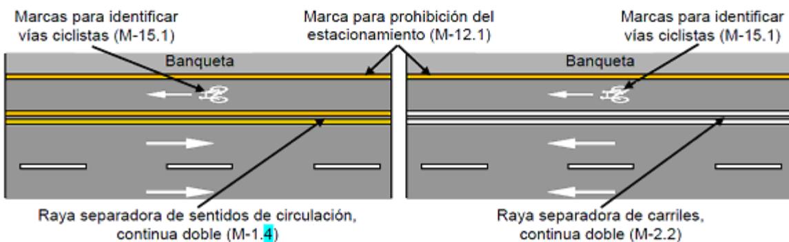
FIGURA 19.- Marcas para delimitar vías ciclistas
