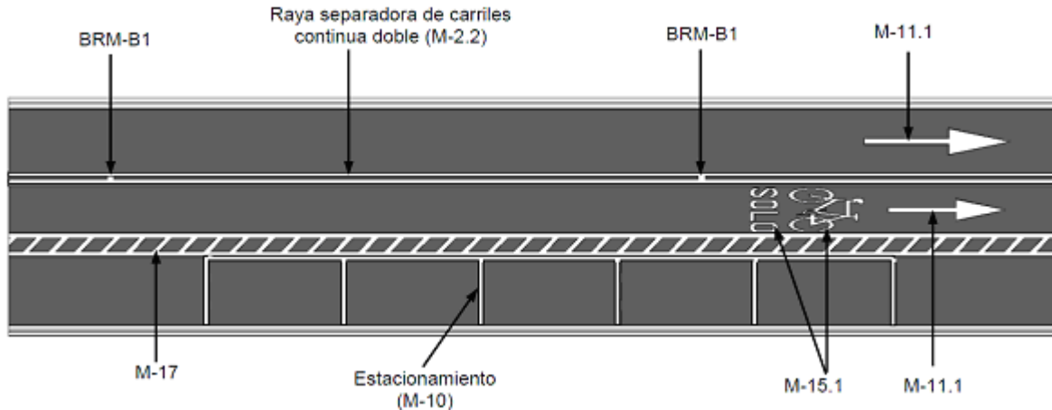
FIGURA 21.- Rayas de protección al ciclista (M-17)
