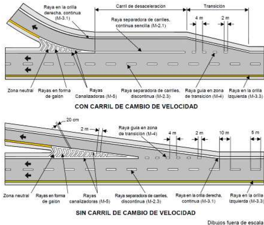
FIGURA 7.- Rayas separadoras de carriles, rayas guía en zonas de transición, rayas canalizadoras y rayas en la orilla del arroyo vial
