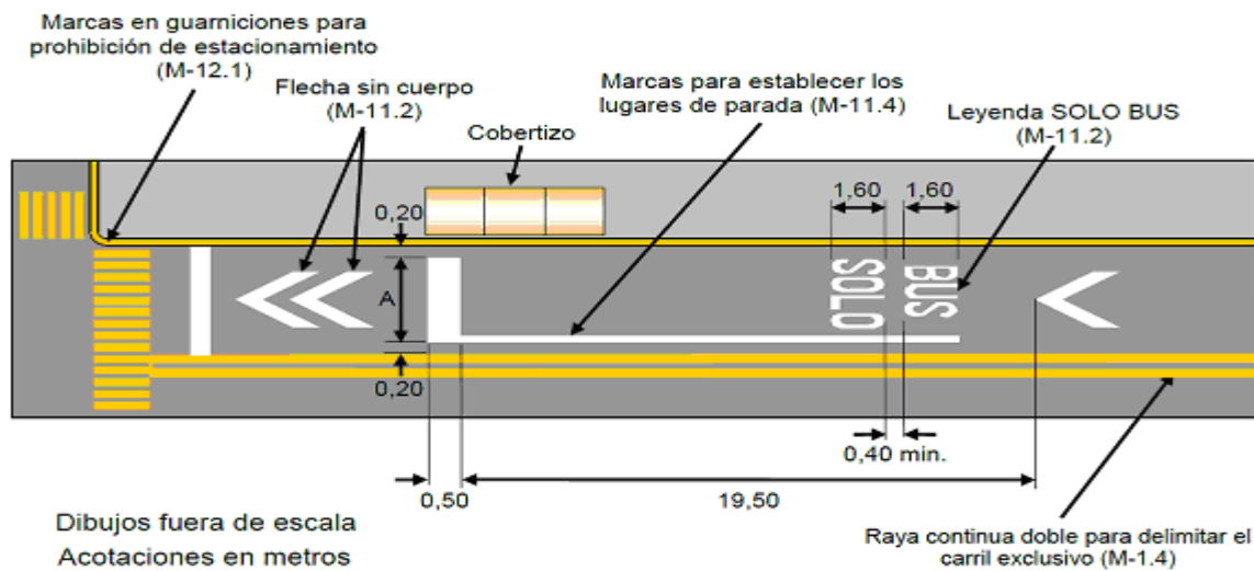
FIGURA 15.- Marcas para establecer lugares de parada en un carril en contrasentido
