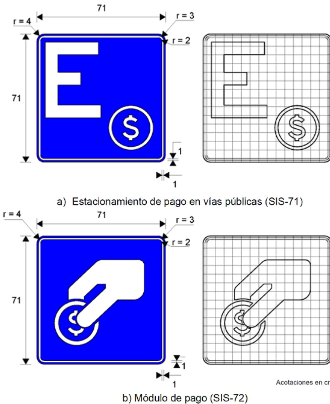
FIGURA 25.- Señales de servicio: estacionamiento de pago en vía pública (SIS-71) y módulo de pago (SIS-72)
