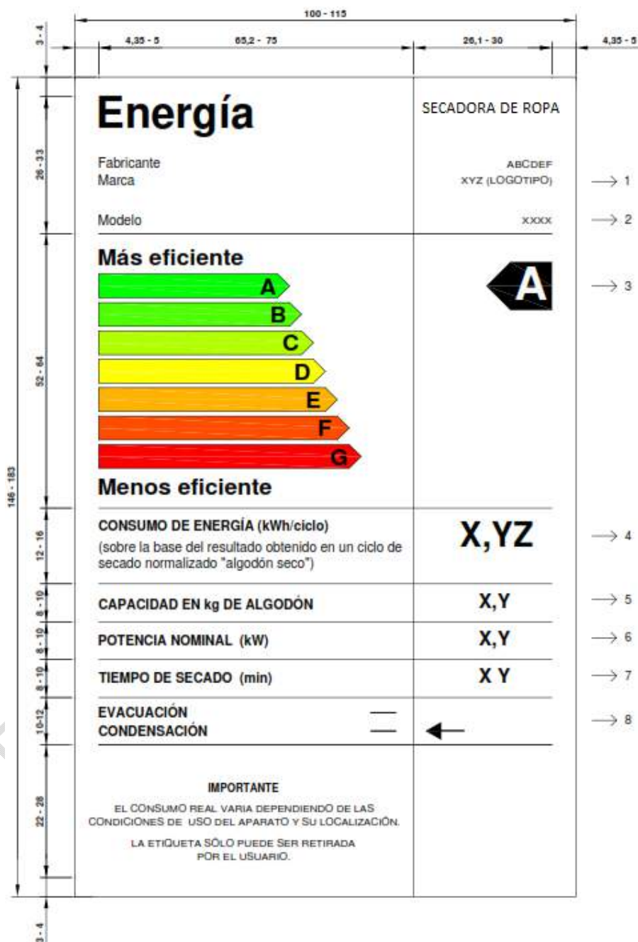
FIGURA 1. Forma, dimensiones e identificación de los campos de la etiqueta de eficiencia energética
