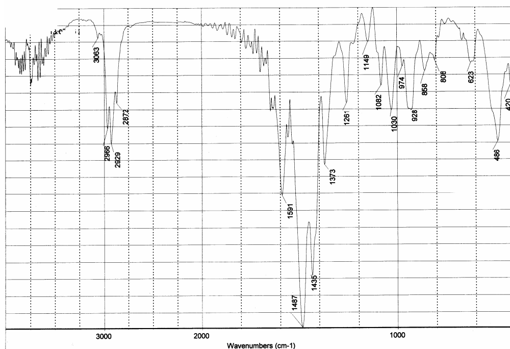
图1 烯草酮标样的红外光谱图
