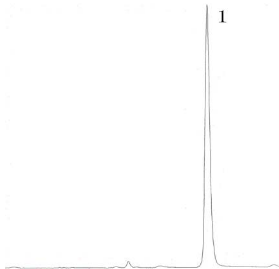
图2 烯草酮原药的正相高效液相色谱图
