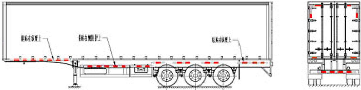
图 A.6 帘布式半挂车
