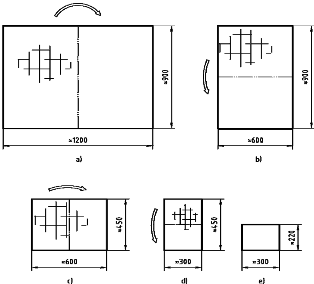
图F.1 标准测试包的折叠和组装
