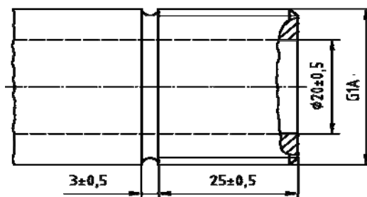
图 2 温度连接器
