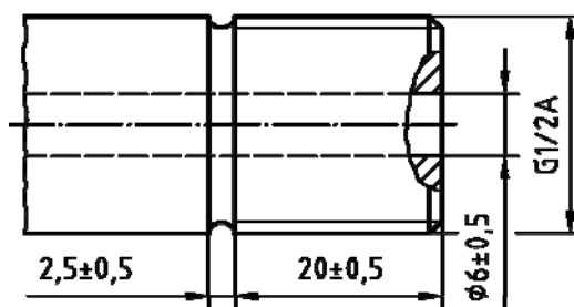
图 1 压力连接器
