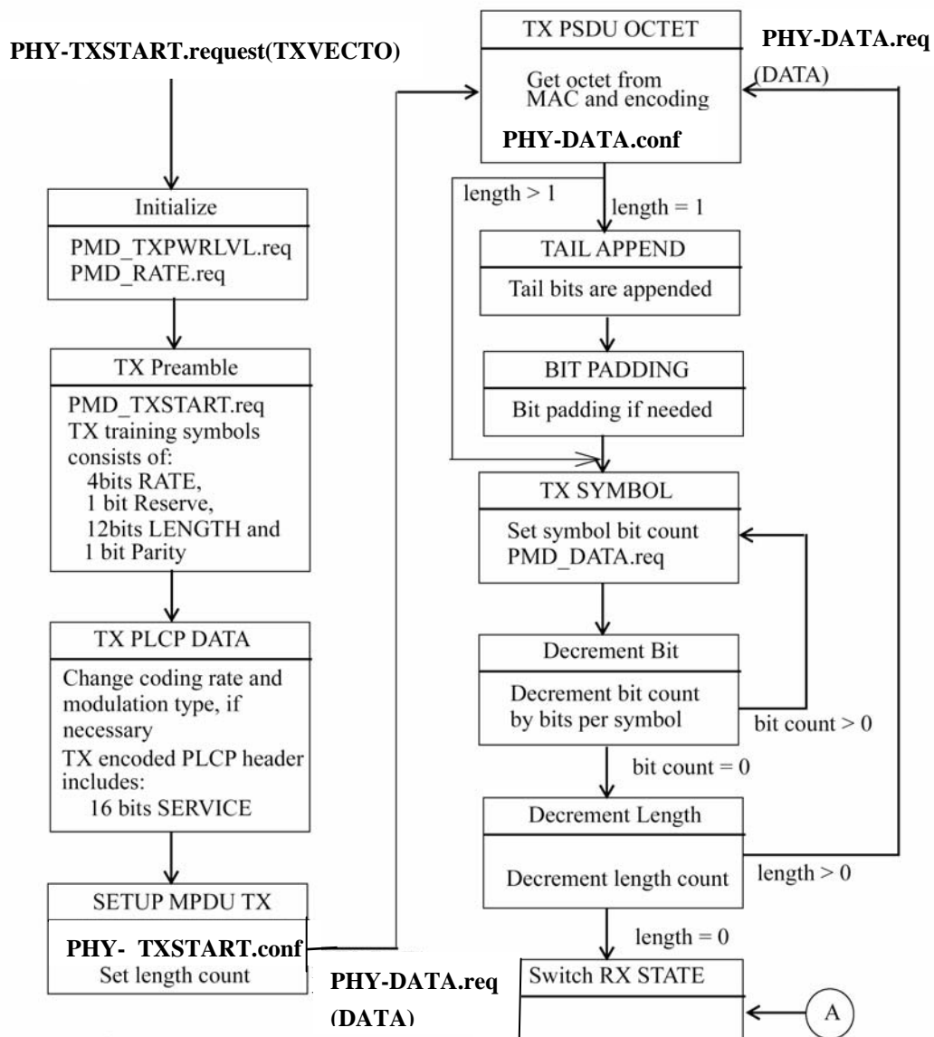
图 17 PLCP 发射状态机
