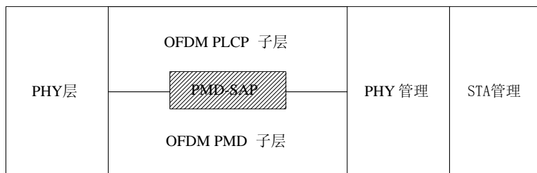
图 20 PMD 层参考模型
