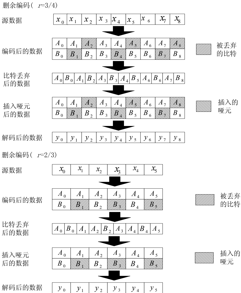
图9 比特丢弃及插入过程举例 ( r = 3/4, 2/3 )
