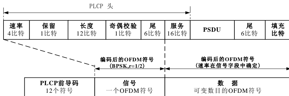
图 1 PPDU 帧格式
