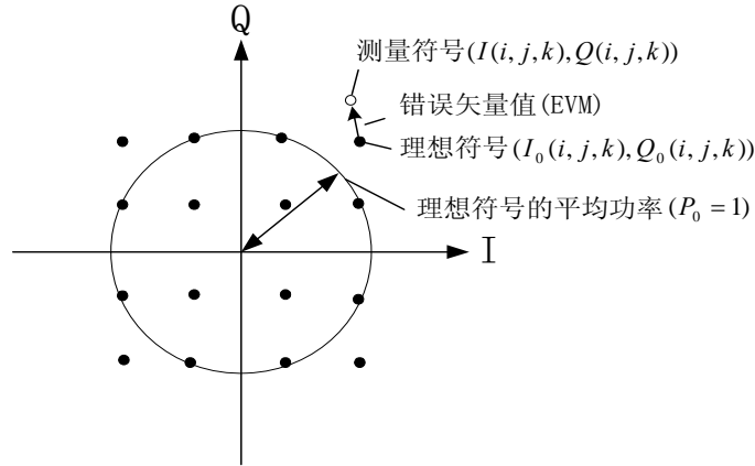
图 15 星座图错误
