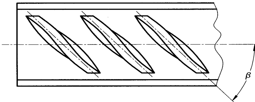
Figura B.1 - Angulos de los resaltes
