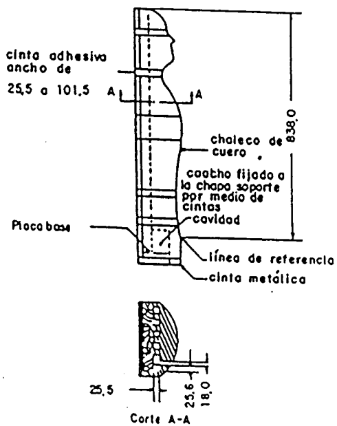
FIG. 4 - PERFIL DEL BLOQUE
