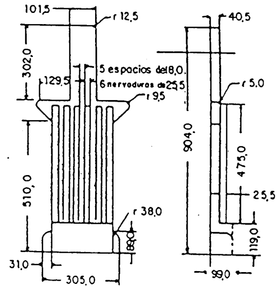
FIG. 2 - ALMA DEL BLOQUE
