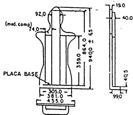
FIG. 3 - CHAPA SOPORTE
